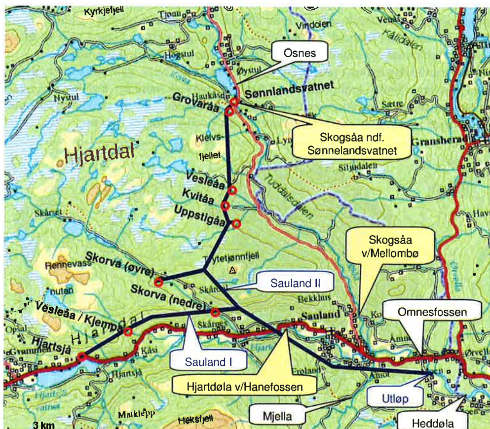
Fig. 2 Kartskisse over utbyggingen. Tunnelene er skissert med blått og inntakspunktene er markert med røde sirkler. Målestedene for vanntemperatur som er plottet i denne rapporten er markert med gul bakgrunn, og stasjonsnavnene er hentet fra NVEs database. Således er Sønnelandsvatnet det samme som Sønderlandsvatn, og Hanefossen det samme som Hanfoss.
