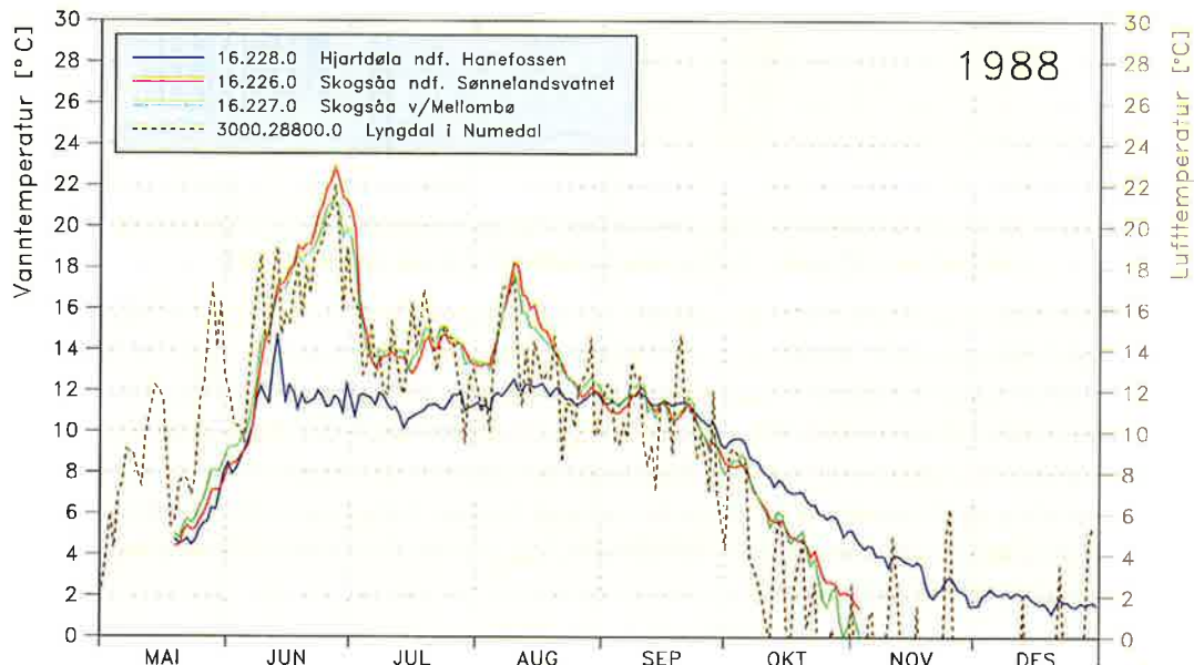
Fig. 5 Vanntemperaturen i Skogsåa nedenfor Sønderlandsvatn (rød strek) og 1.5 km oppstrøms samløpet med Hjartdøla (v/Mellombø, grønn strek). Samtidig vises vanntemperaturen i Hjartdøla ved Hanfoss (blå strek) og lufttemperaturen i Lyngdal (striplet brun strek) som antas å være representativ for området. Alle dataene er døgnmidler.
