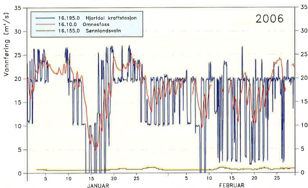
Fig. 3 Driftsvannføringen i Hjartdøla kraftverk, vannføringen i Heddøla ved Omnesfossen, og vannføringen i Skogsåa nedenfor Søndrelandsvatn i januar og februar 2006.
