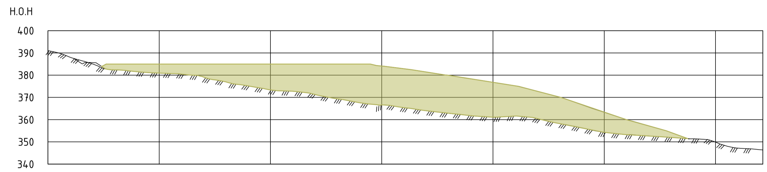
Snitt A-A 1:1000
